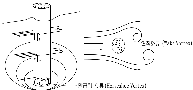
【그림 3.2.15】 원형기초의 국부세굴
