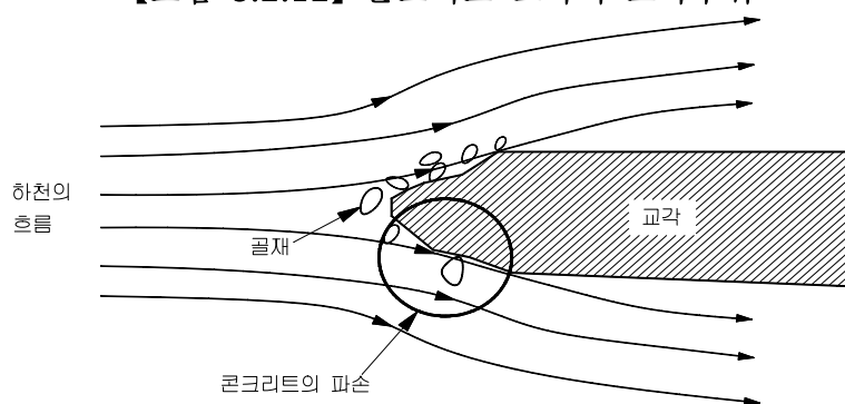
【그림 3.2.13】 유수에 의한 콘크리트 교각의 침식
