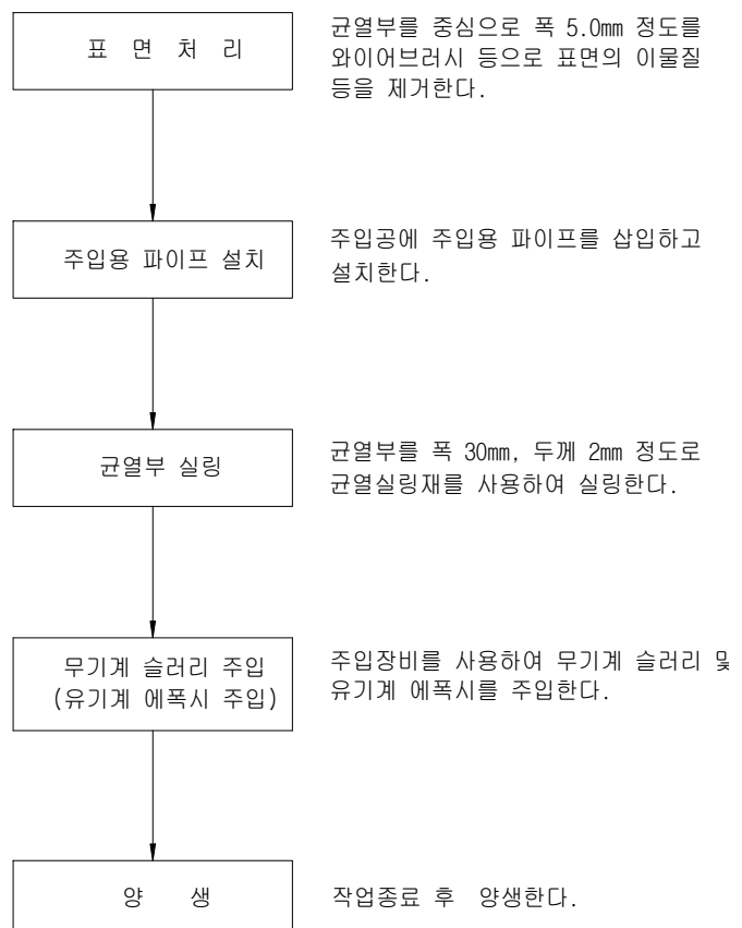
【그림 5.3.2】 균열 보수공법 개요도
