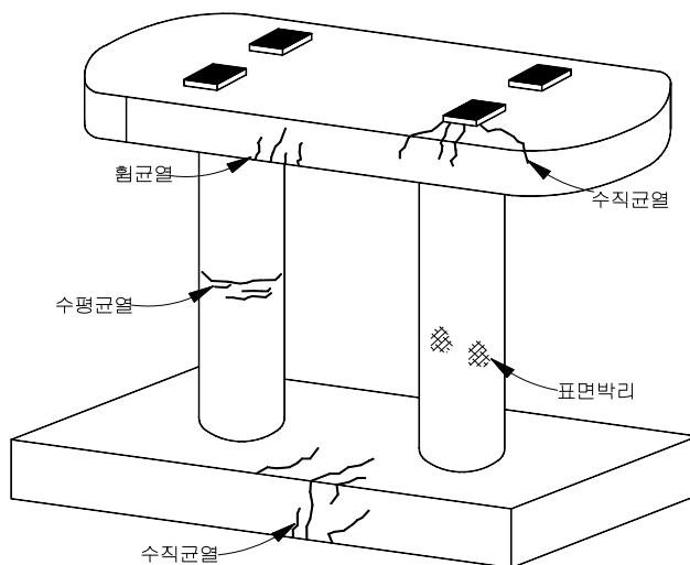
【그림 3.2.12】 콘크리트 교각의 조사부위
