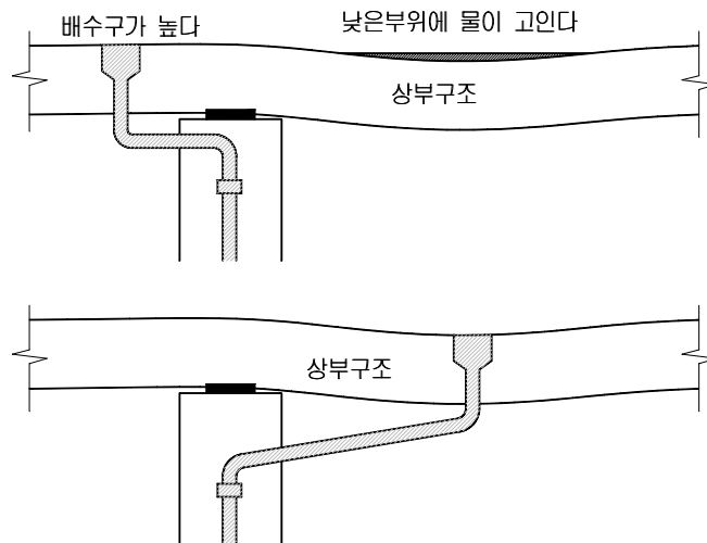
【그림 3.2.21】 배수구 물고임
